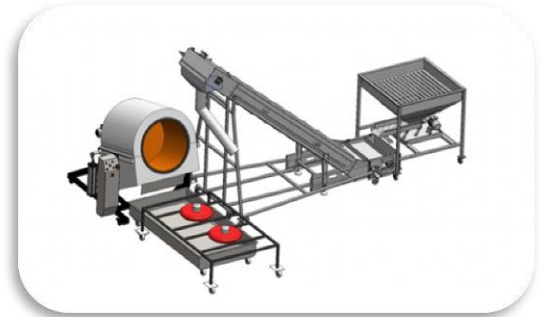
ОХЛАЖДАЮЩИЙ ПОДДОН
